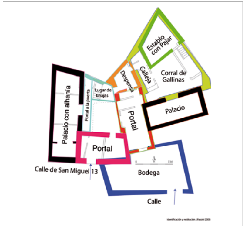
Figura 5. Interpretación de la Planta de Estado Actual del inmueble (Izquierda), basada en la documentación del siglo XV del cabildo de la Catedral de Toledo. A la derecha se muestra la distribución de las distintas estancias que componían el inmueble en el Siglo XV, realizada por Jean Passini (PASSINI, Jean, Casas y casas principales urbanas. El espacio doméstico de Toledo a fines de la Edad Media, UCLM, Fundación Toledo y otros, 2004)
